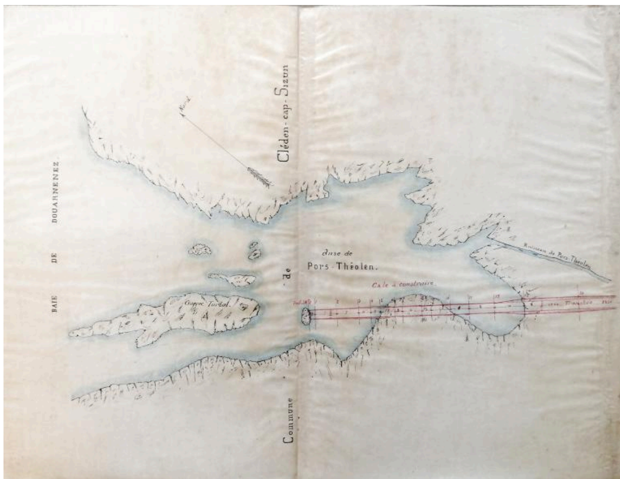
Anse de Pors Théolen, construction d'une cale. Plan général. Reproduction plan des Ponts et Chaussées 31/01/1883.
