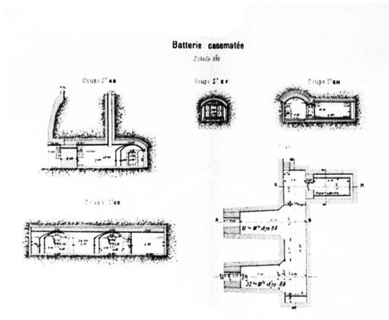
Plans et coupes des batteries casematée et à tir rapide du Minou, 1893 : détail de la batterie casematée (Direction d'Artillerie du génie de Brest, colonel directeur d'Artillerie Collomb)
