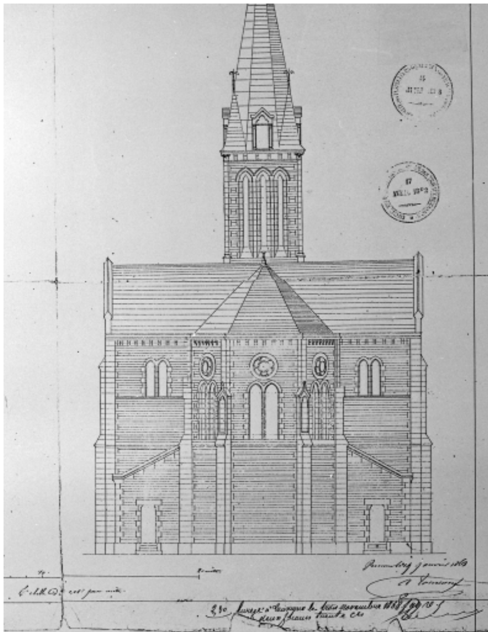
Elévation du chevet de l'église
