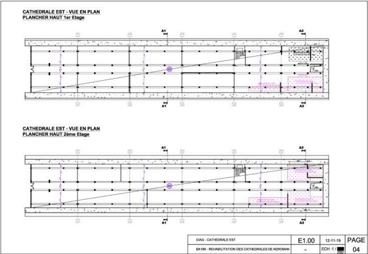
Vue en plan : plancher haut premier étage et plancher haut deuxième étage, 2019 (Projet de réhabilitation des cathédrales de l'aire de réparation navale de Lorient-Keroman)
