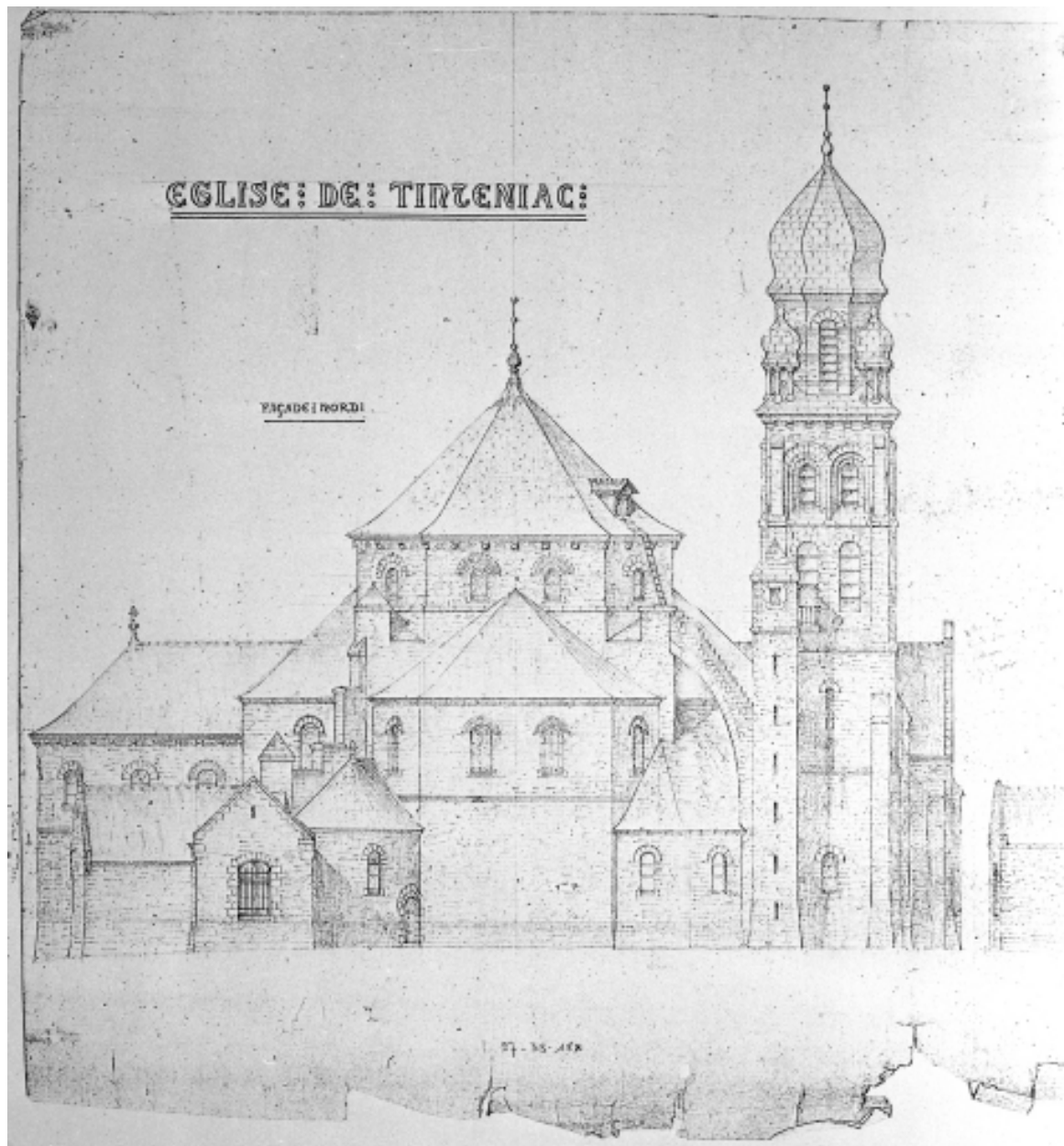
Projet pour l'église de Tinténiac : élévation de la façade nord, dessin par Arthur Regnault
