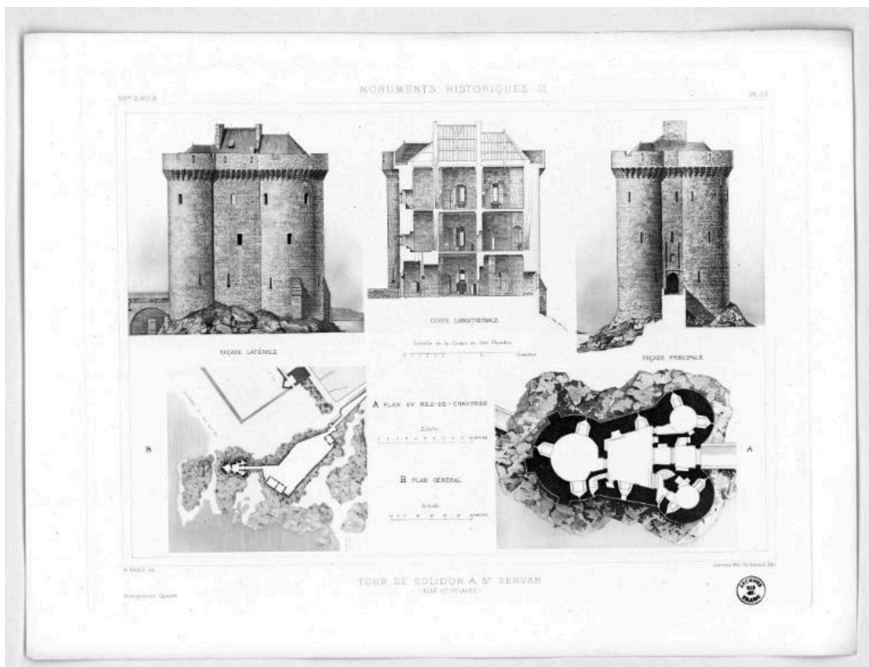
Monuments historiques II. 14e siècle. Planche 53. Tour de Solidor à Saint-Servan (Ille-et-Vilaine). Façade latérale. Coupe longitudinale. Façade principale. Plan du rez-de-chaussée. Plan général. (Albert Ballu ; héliogravure Chauvet)
