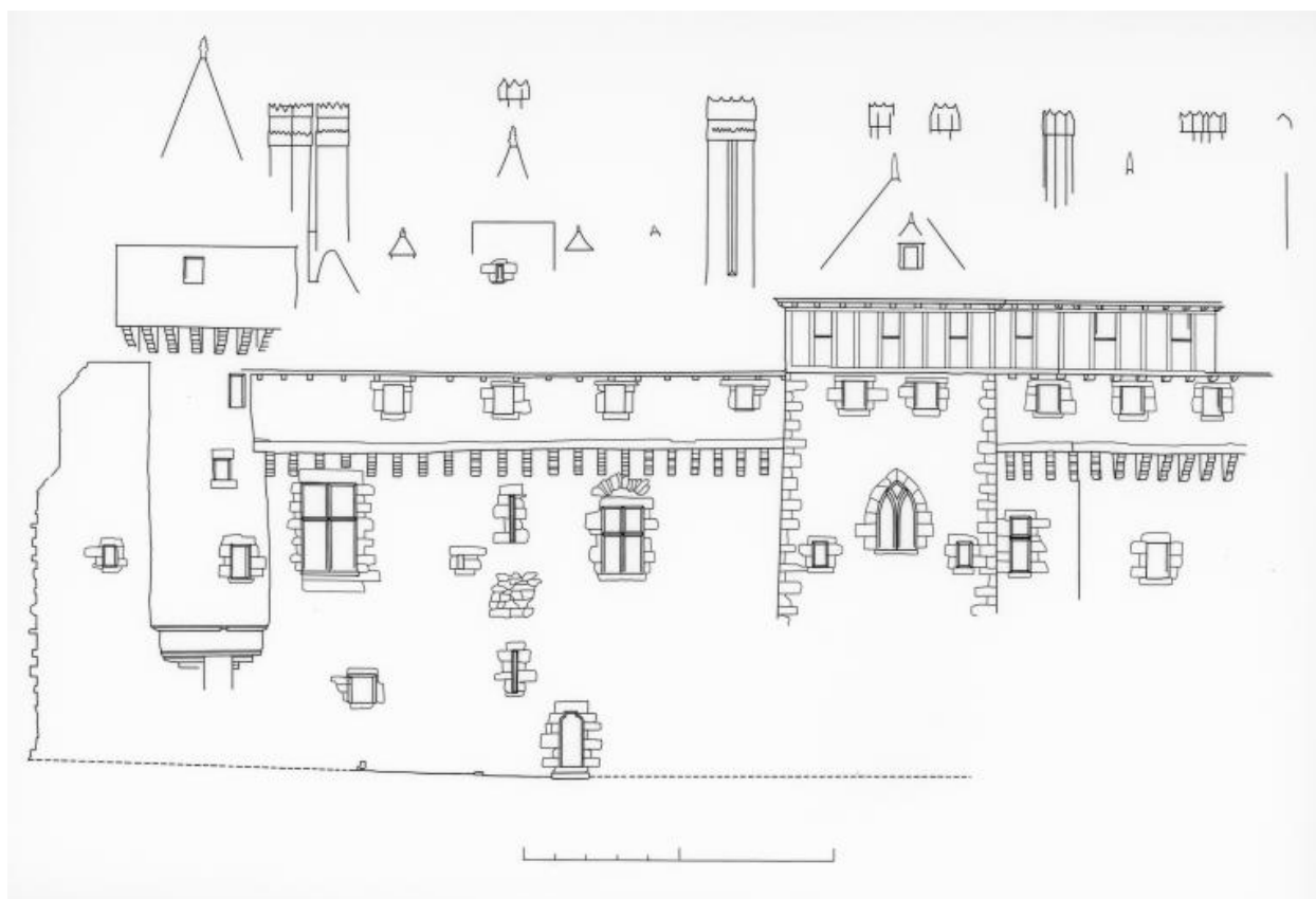
Élévation postérieure côté Trieux, relevé par photogrammétrie, 1974
