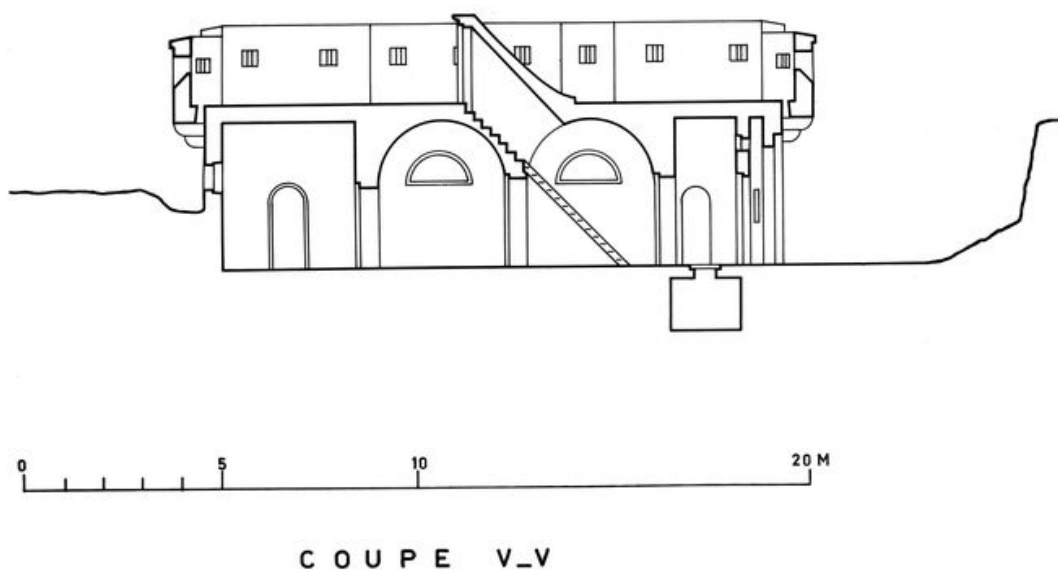
Coupe V-V du corps de garde crénelé n° 3 du bourg de Roscanvel
