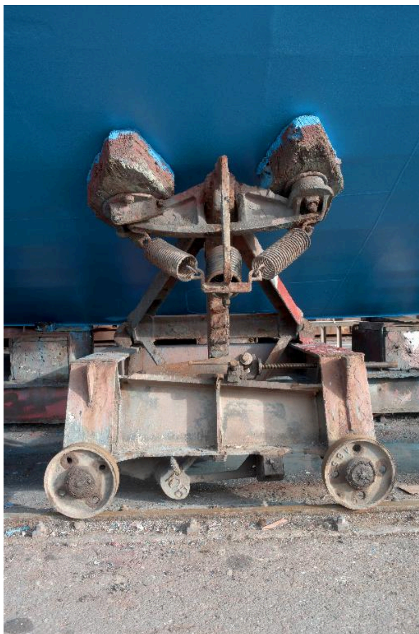
Ber, patins, vue rapprochée
