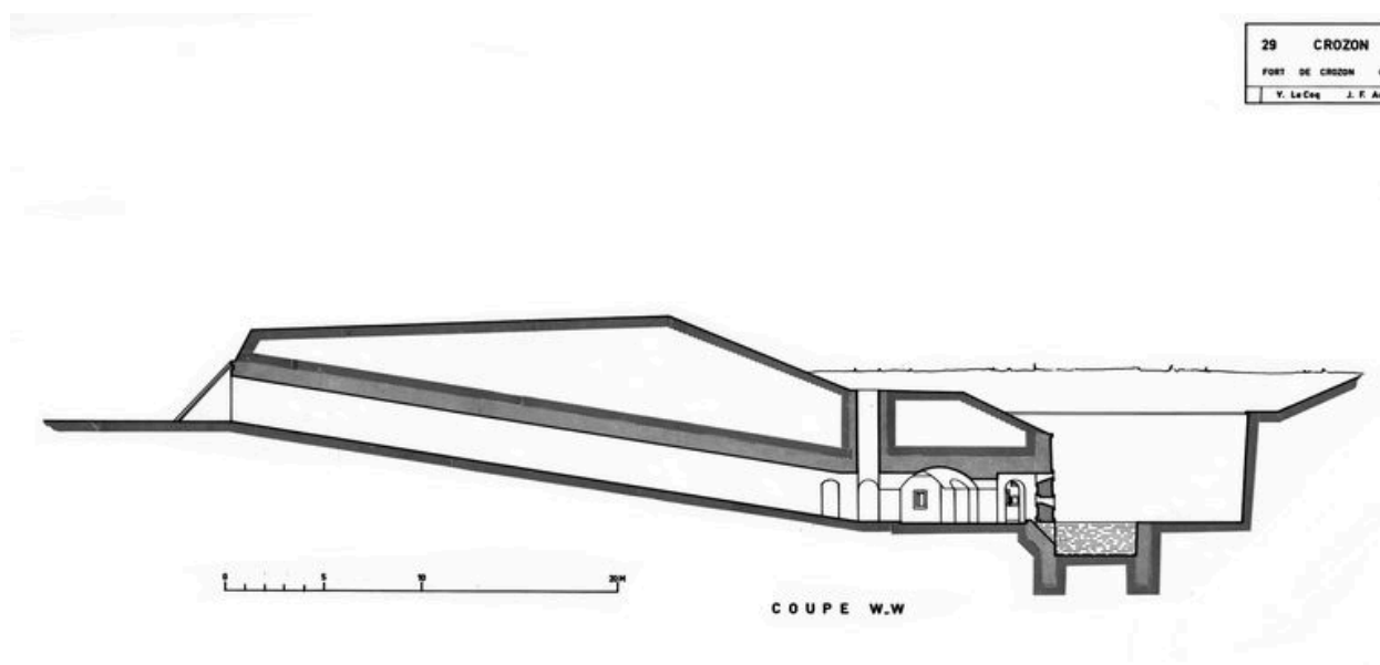
Coupe W-W de la caponnière Ouest (D) (Lecoq)
