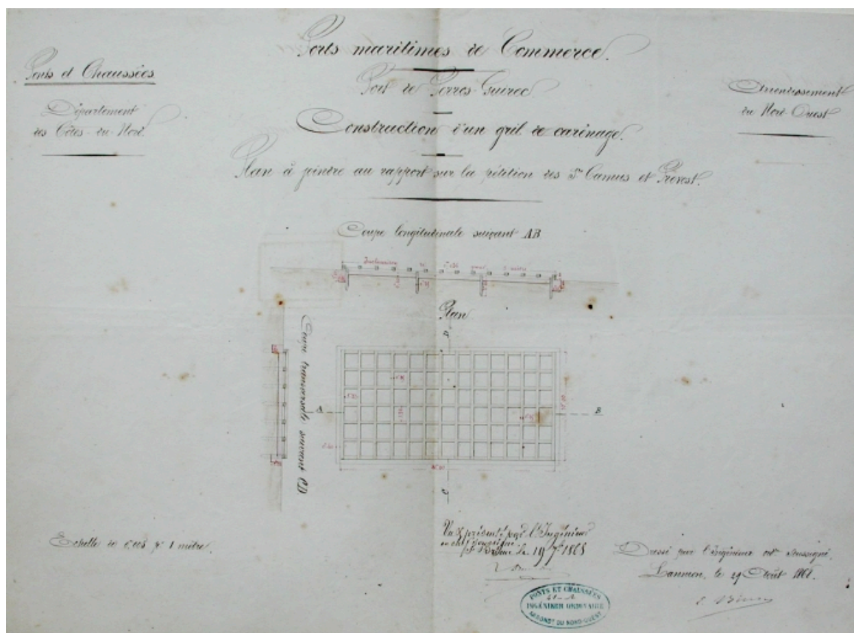
Plan : projet d'un gril de carénage en 1868 (AD 22)
