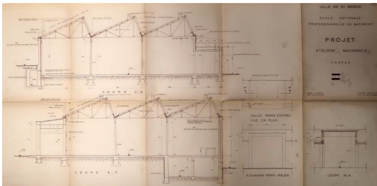
Ateliers - Bâtiment E. Coupes. Yves Moignet, architecte, 1960.
