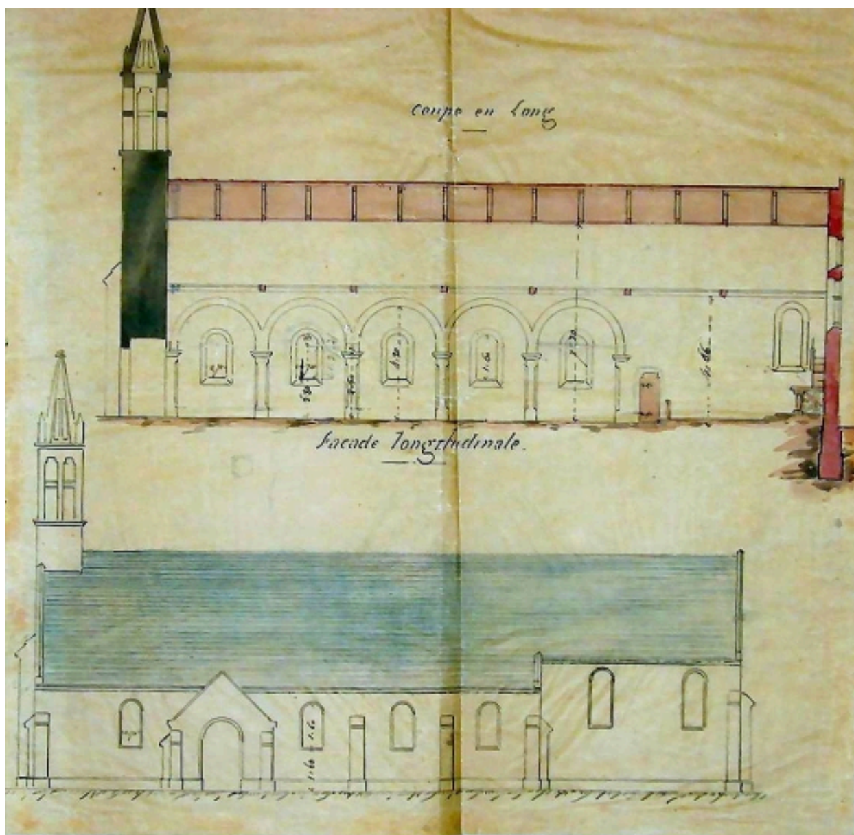
Locunolé, église paroissiale Saint-Guénohé : projet (coupe longitudinale et élévation sud) réalisé, par Joseph Bigot, 1863 (A. E. Quimper, 8 L fonds Bigot), reproduction de 2004
