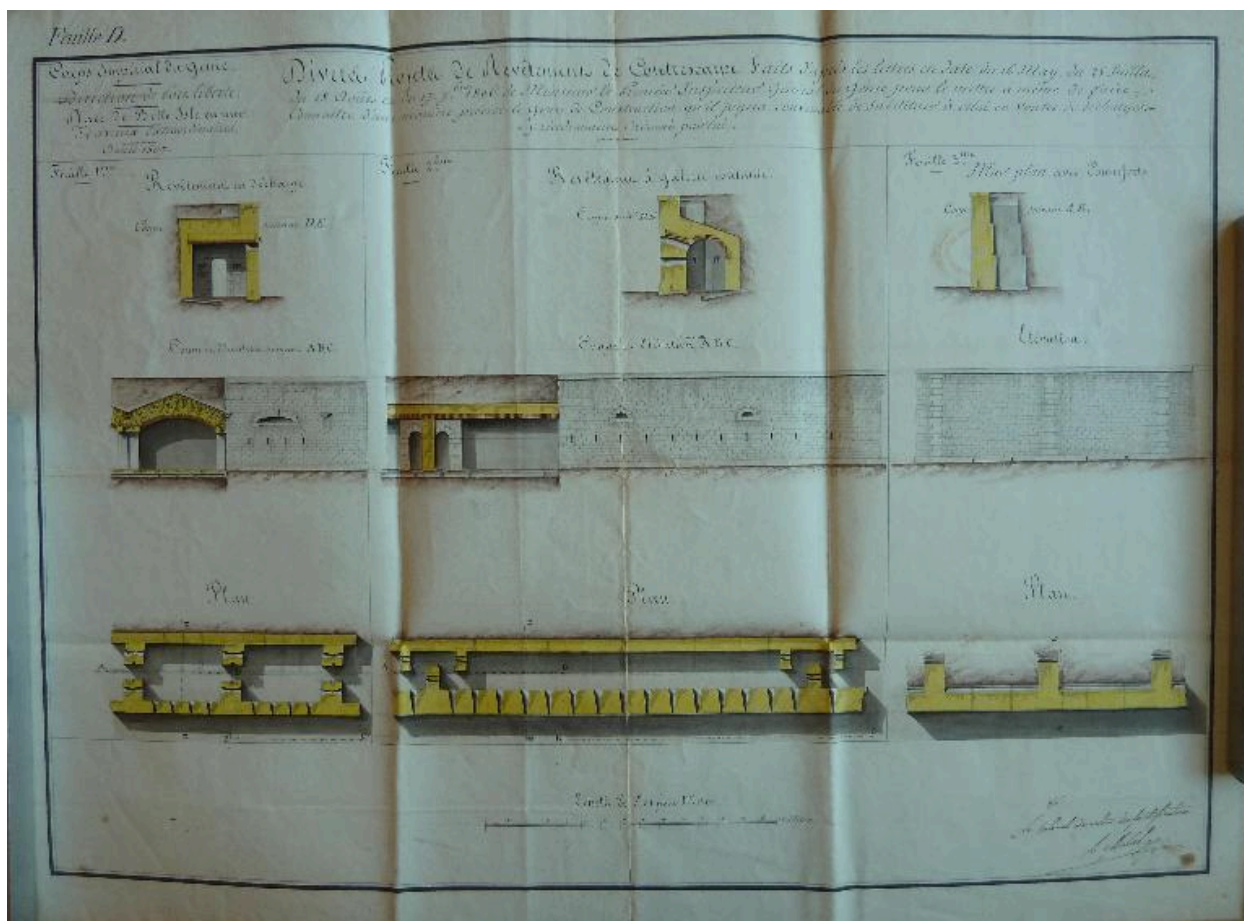
1 VH 286. Place de Belle-Ile-en-Mer, divers projets de revêtement de contrescarpe, 2 novembre 1807.
