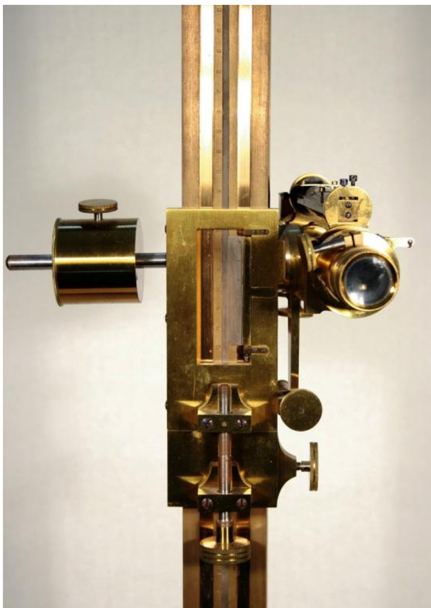
Détail du cathétomètre – Pesanteur-Mécanique-Mesure (E. Ducretet)
