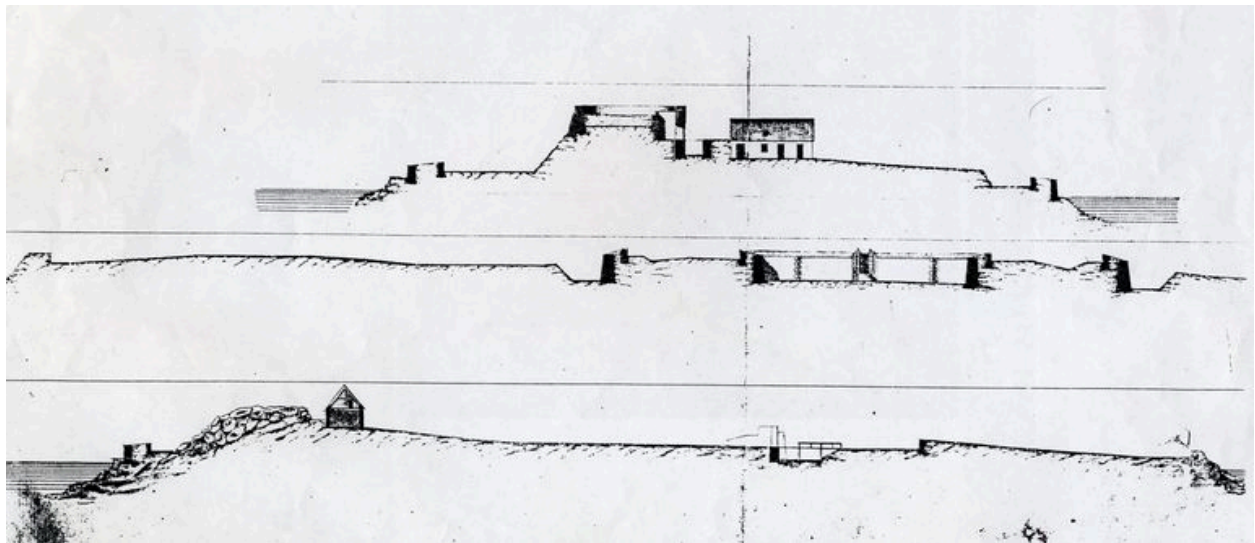
Coupes du fort Cézon, milieu du 19e siècle, auteur inconnu, Service historique de la Défense, Brest, série Z génie, E59 (Yann Le Nestour, Florence Fröhlig - association Cézon, document n° 12)
