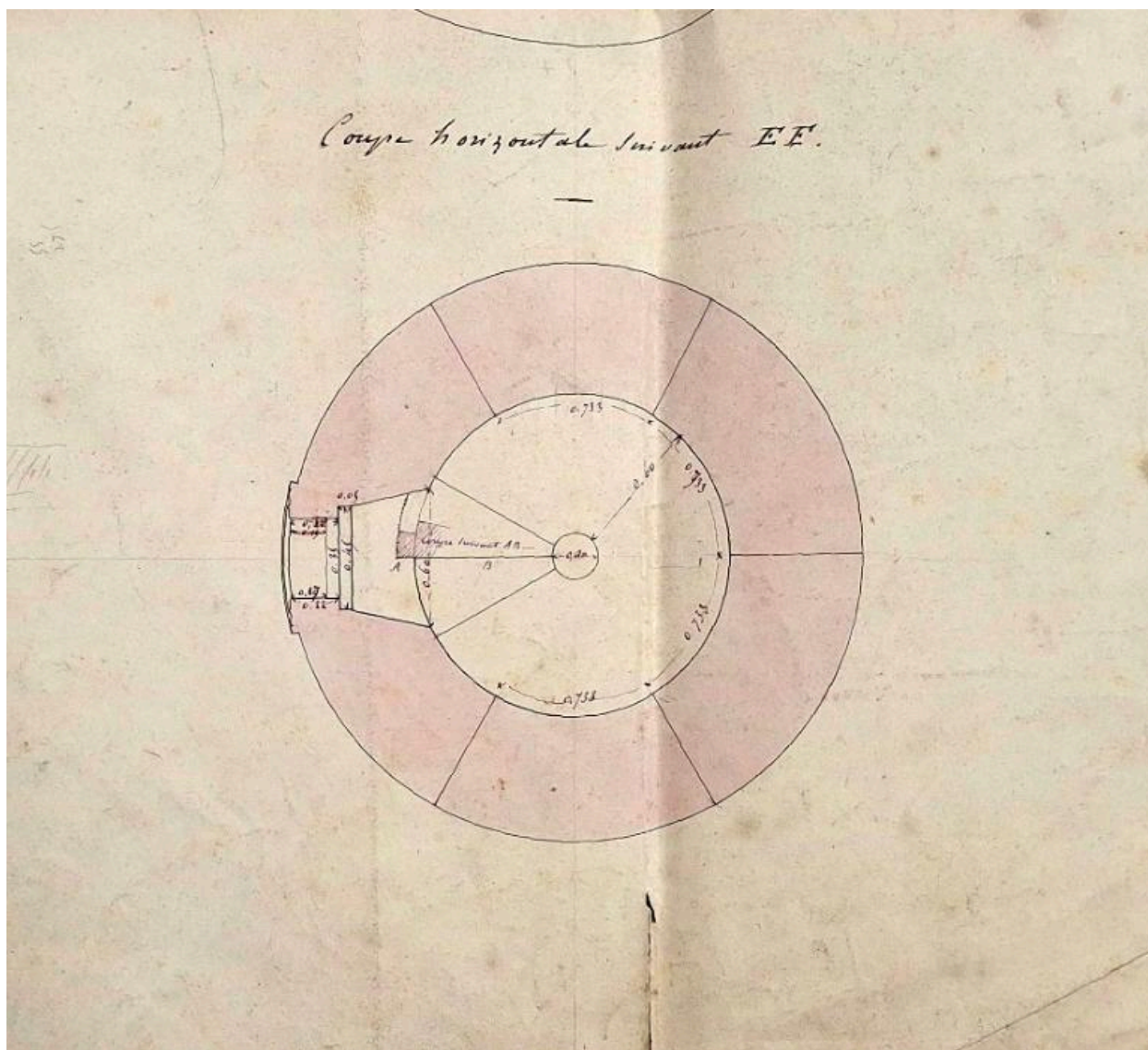
Coupe horizontale du phare de la pointe de l'Aigle (18 novembre 1855)
