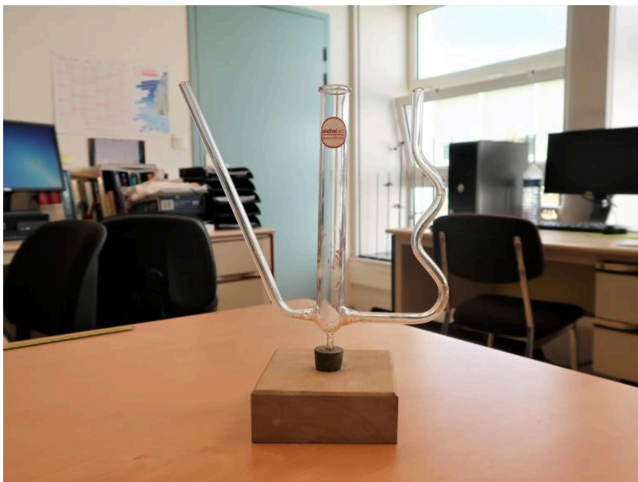
Appareil des vases communicants - Hydrostatique-Hydrodynamique (Didalab)
