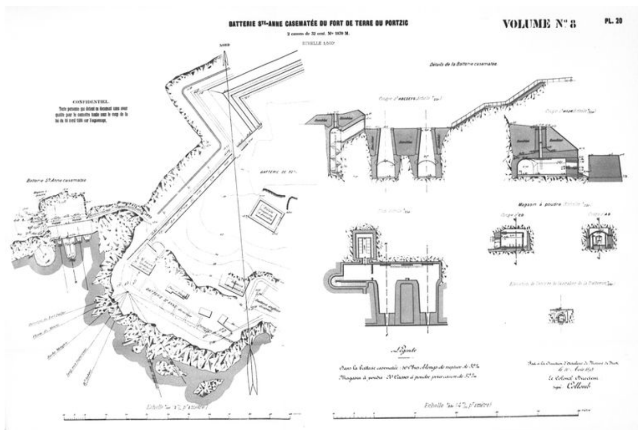
Plan et coupes de la batterie casematée du fort de terre du Portzic, 1893 (Direction d'Artillerie du génie de Brest, colonel Directeur d'Artillerie Collomb)
