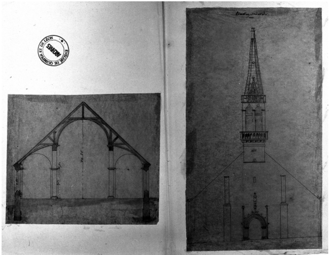
Châteaulin, église paroissiale Saint-Idunet : Elévation et coupe, Joseph Bigot, 1867. (A.E. Quimper)
