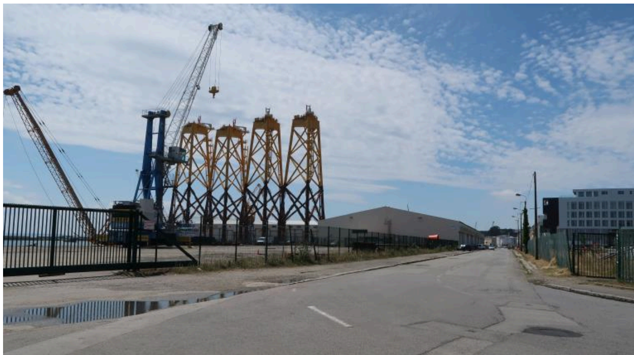
Fondations du parc éolien de Saint-Brieuc : 4 jackets de 75 m de haut
