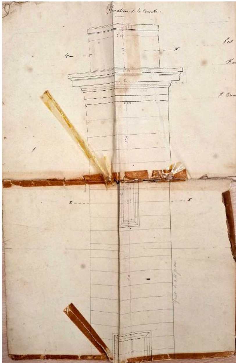
Plan du phare de la pointe de l'Aigle (18 novembre 1855)
