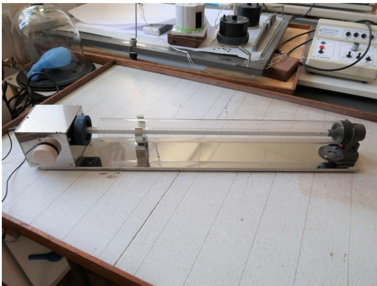
Tube de Kundt à sorties analogiques - Acoustique-Vibration (Jeulin)
