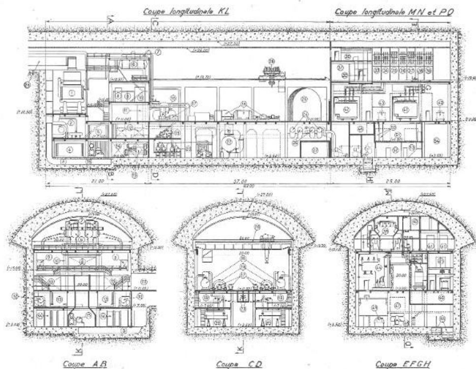
Fig. 5. — Alvéole principale de la centrale électrique souterraine du Portzic.
