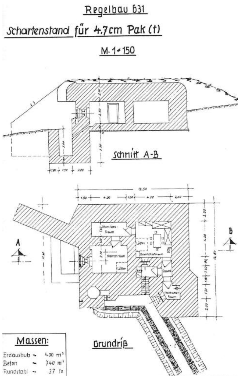
Plan d'un bunker - casemate de type 631 (Schartenstand für 4,7 cm Pak)
