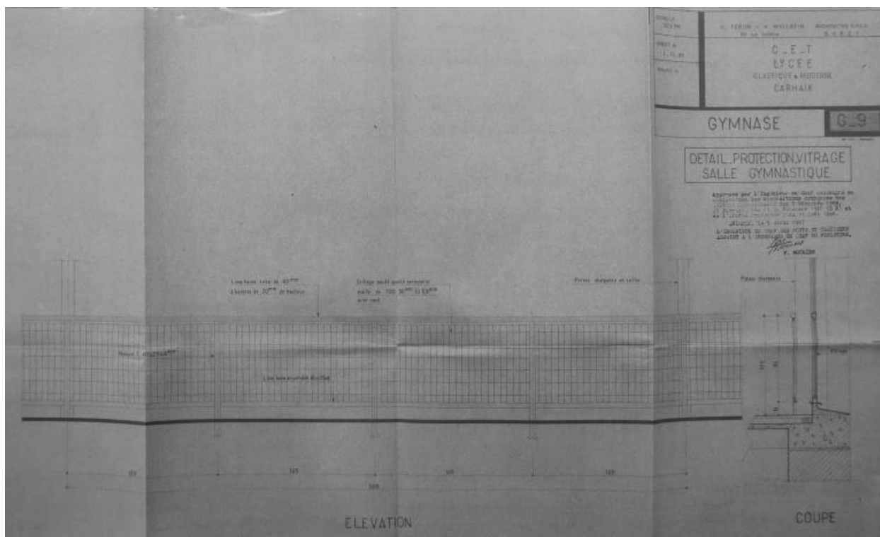
Détail protection vitrage salle de gymnastique. H. Péron et A. Weisbein, architectes, 22/07/1965.
