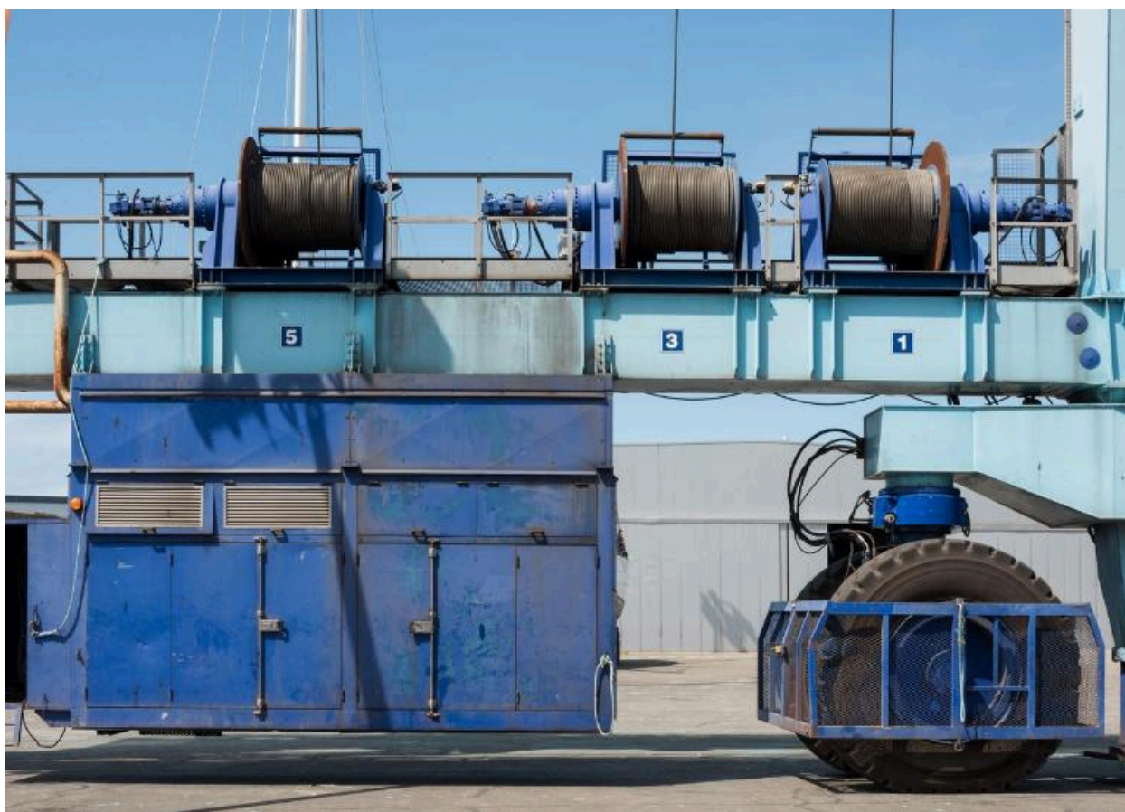
Vue de détail de l'élévateur à bateaux
