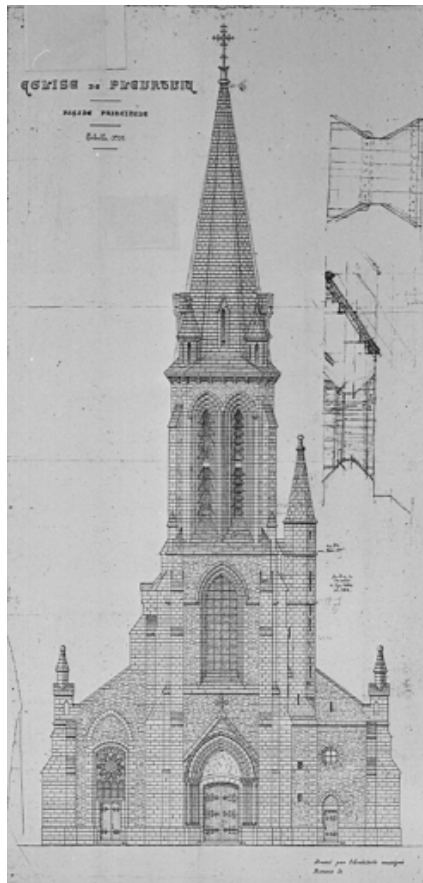
Un projet de façade par A. Regnault
