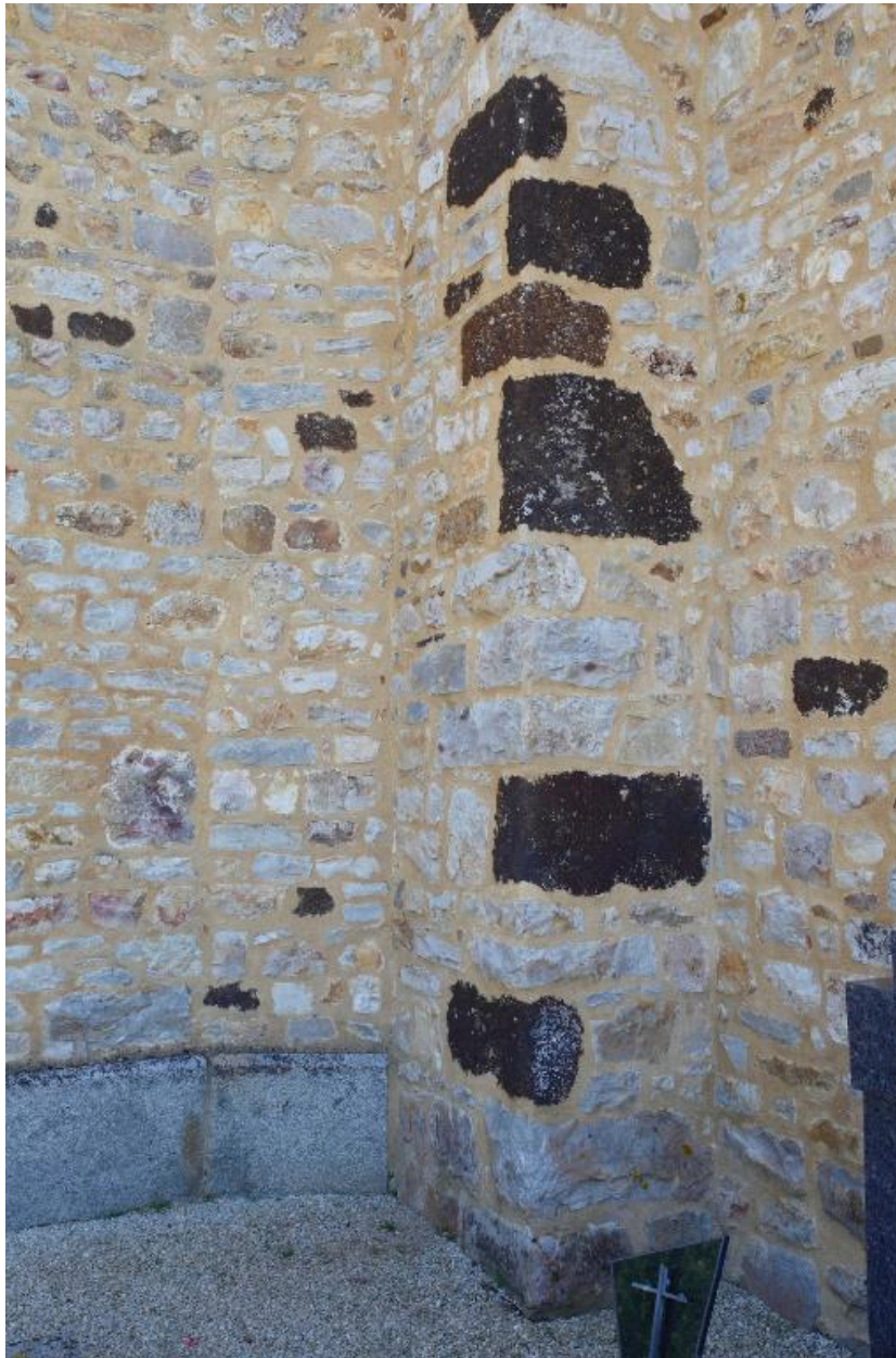
Détail d'un chaînage d'angle
