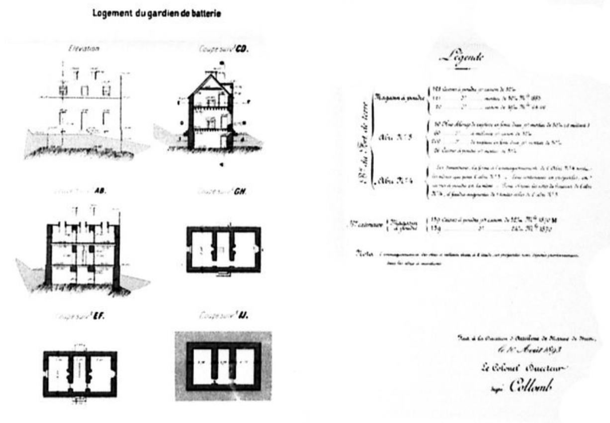
Plan et coupes du logement du gardien du fort du de terre du Portzic, Direction d'Artillerie du génie de Brest, 1893
