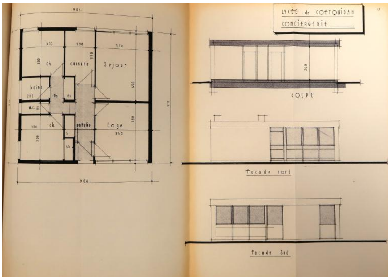
Conciergerie. Plan et élévations.
