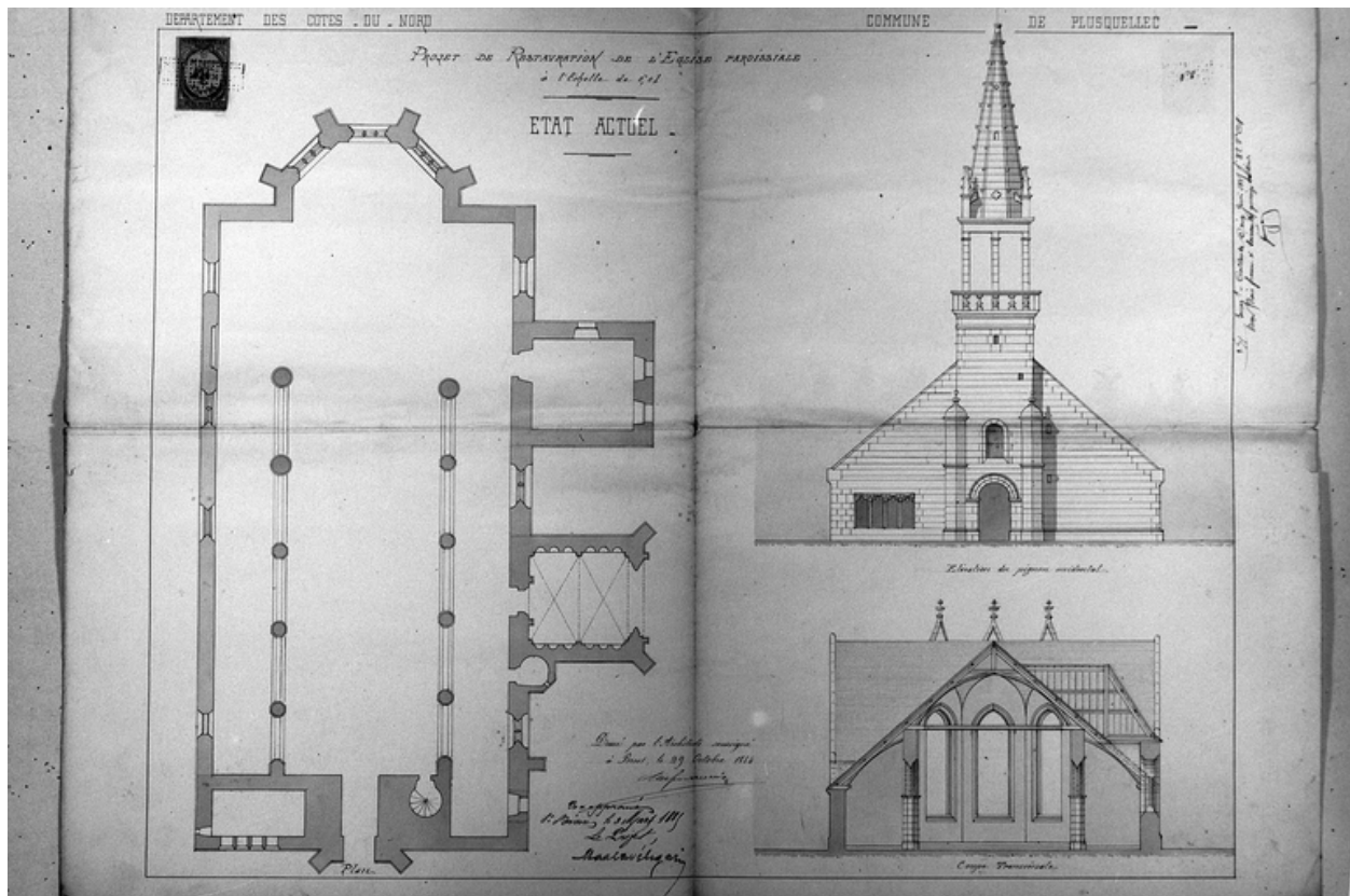
Plan : coupe transversale et élévation de la façade ouest avant restauration
