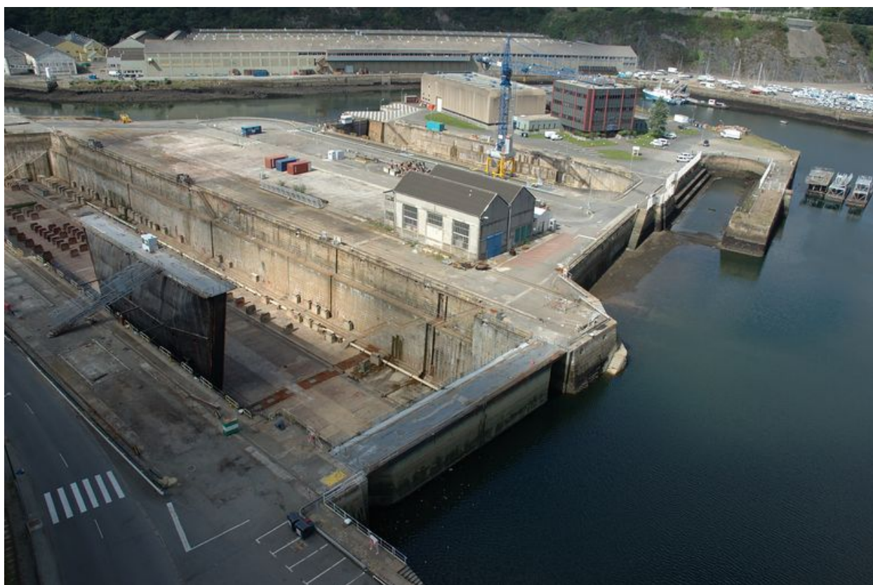
Vue d'ensemble des formes de construction, bassins de radoub actuellement bassins n° 4, 6 et 7 depuis le pont de l'Harteloire
