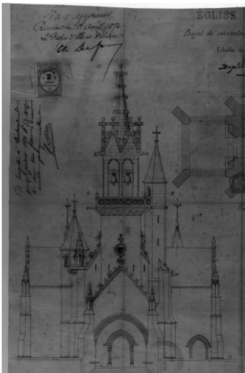
Projet de reconstruction du clocher, vue de face
