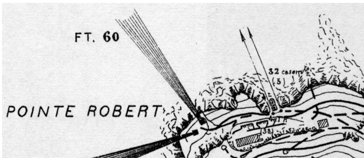
Détail du plan de situation des batteries de Robert et du Stiff : batterie du fort Robert (batterie casematée de 32 cm, projecteur de 90 cm FT, projecteur de 60 cm FT), Atlas des batteries de côte : côte de Brest, 1913, Vincennes
