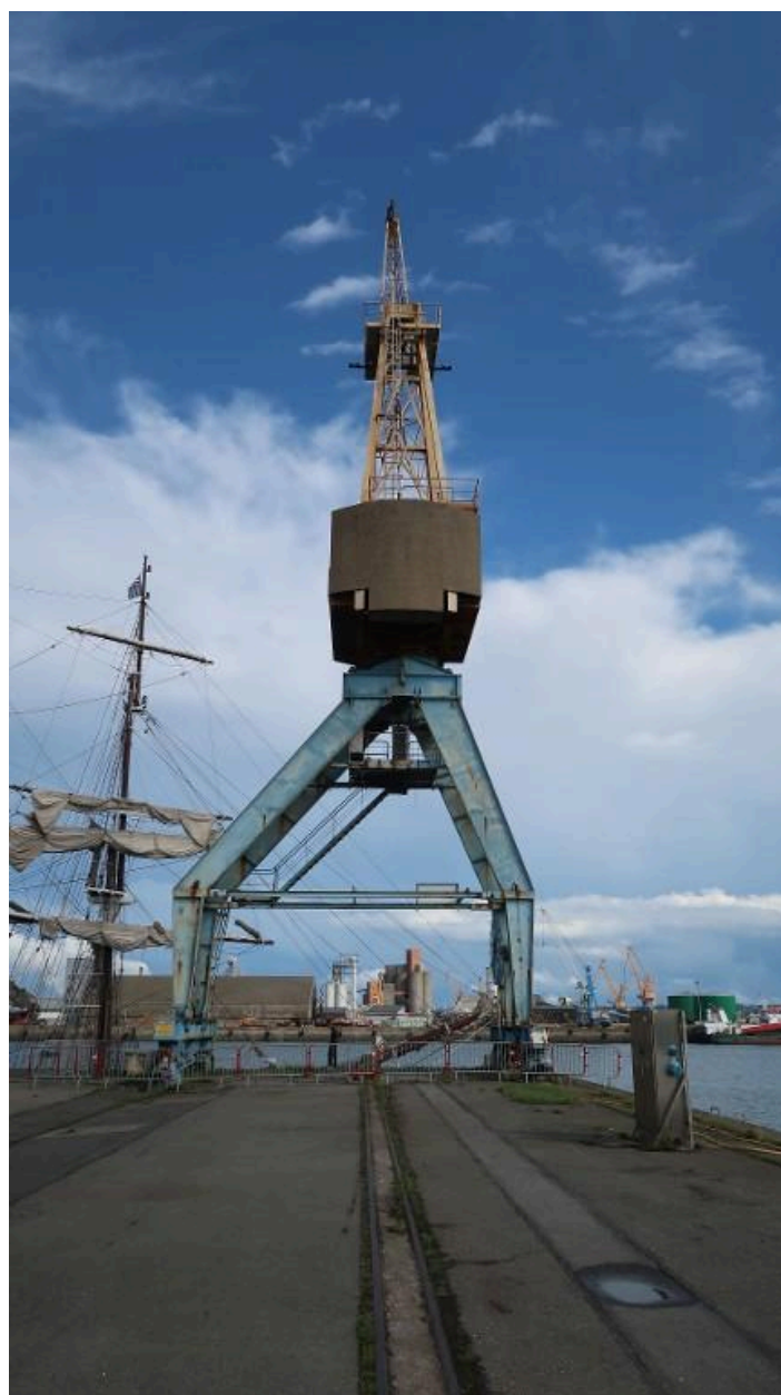
Grue Peiner n°1 située sur le 3e éperon
