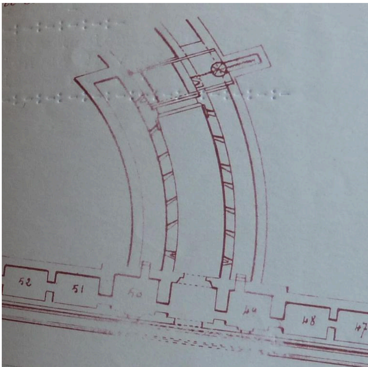
3 V 769. Commission de déclassement et d'aliénation d'ouvrages anciens, 1946-1947, Belle-Île, plan des casemates de contrescarpe et des réduits B et G.
