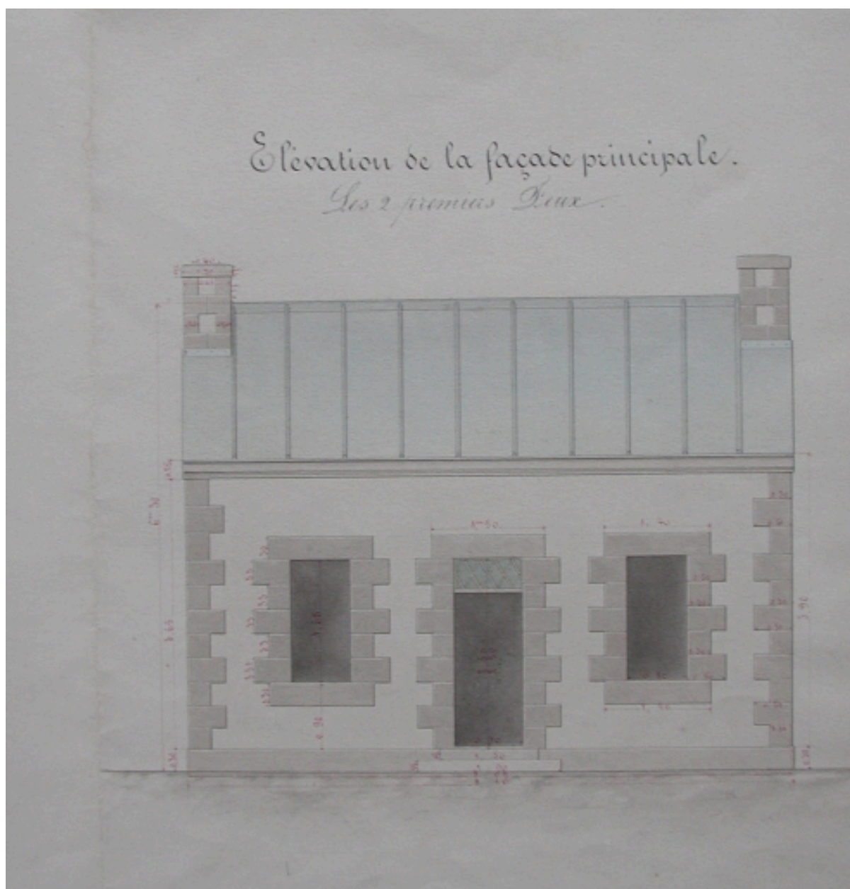
Elévation de la façade principale de la maison-phare, 1857 (AD 22)
