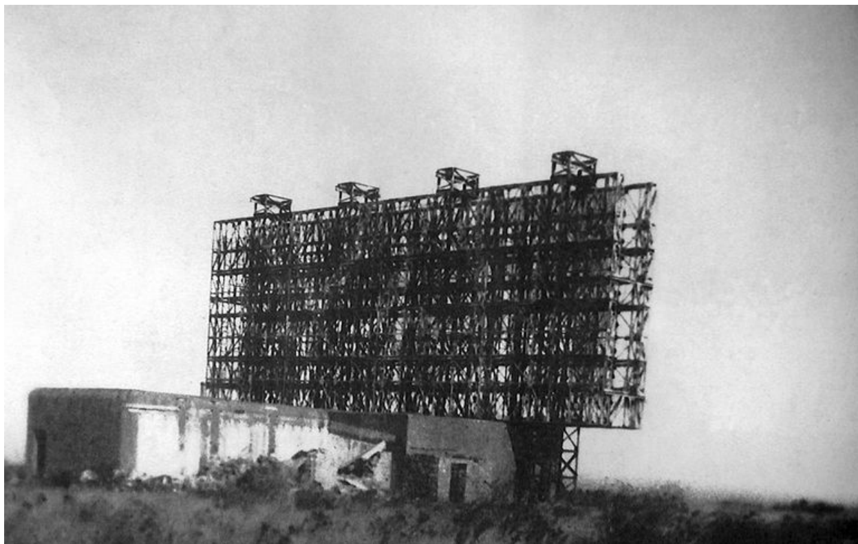
Vue générale du bunker avec son antenne, 1944 (collection : Olivier Doher)
