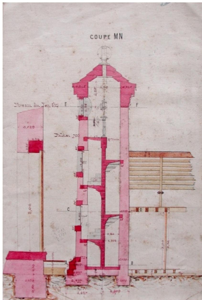
Transformation du feu : dessin en coupe de la tourelle, 1882 (AD 22)
