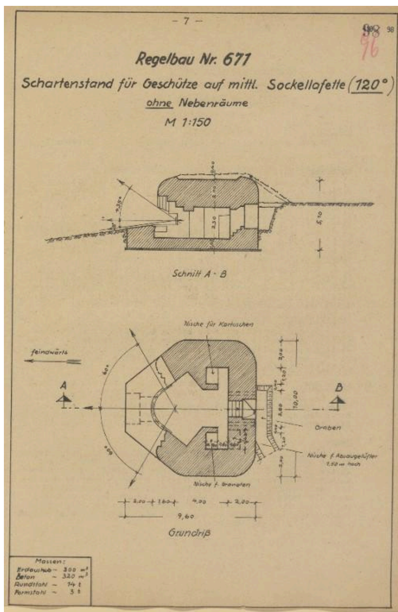
Plan d'un bunker-casemate de type 671 (source : (Bundesarchiv : RH_2_410_0197))
