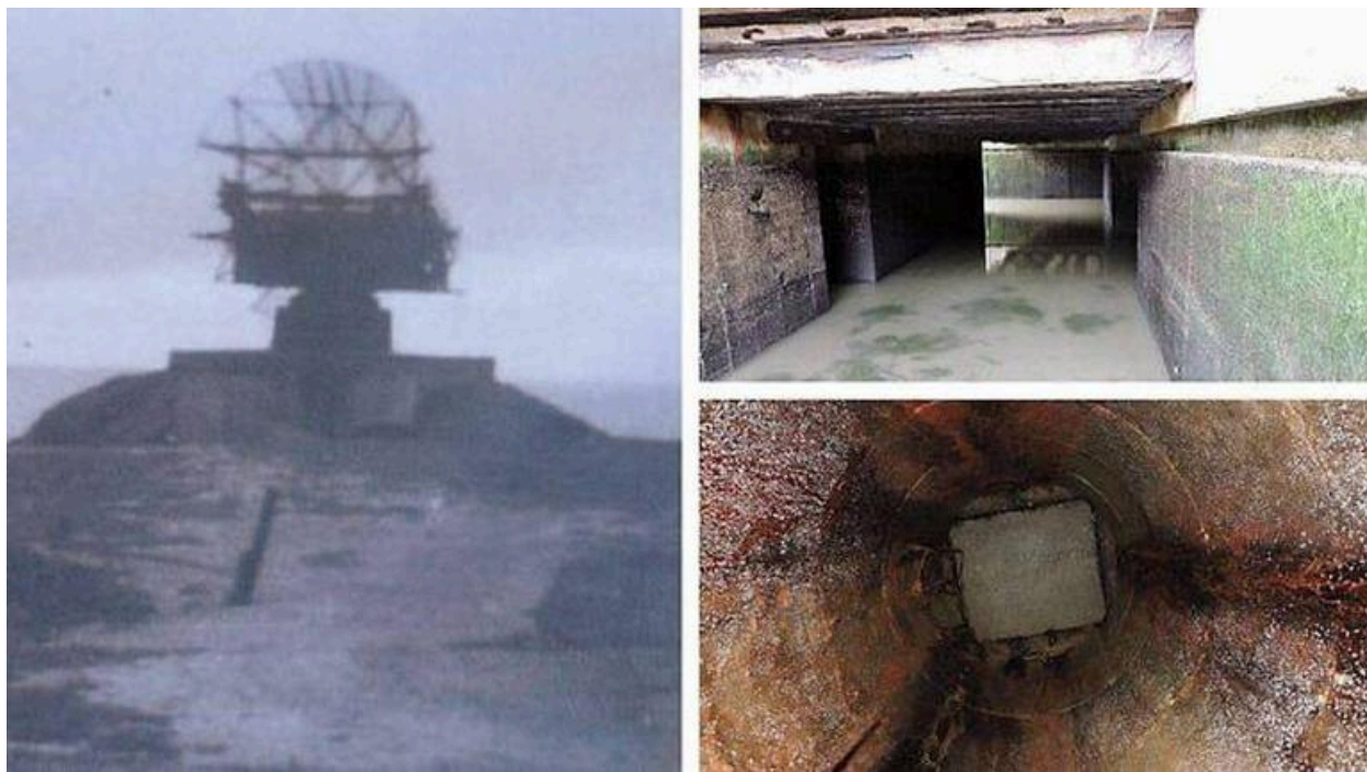
Vue du radar Würzburg See Riese sur son abri (1943) et du bunker V206 (2015), collection Société historique de Belle Île - Jacques Tomine
