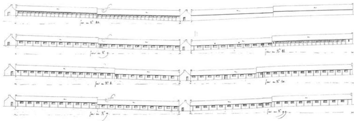
Elévations des établissements maritimes du port de Brest, année 1807. Hôpital du Séminaire, bâtiments n° 7 à 11
