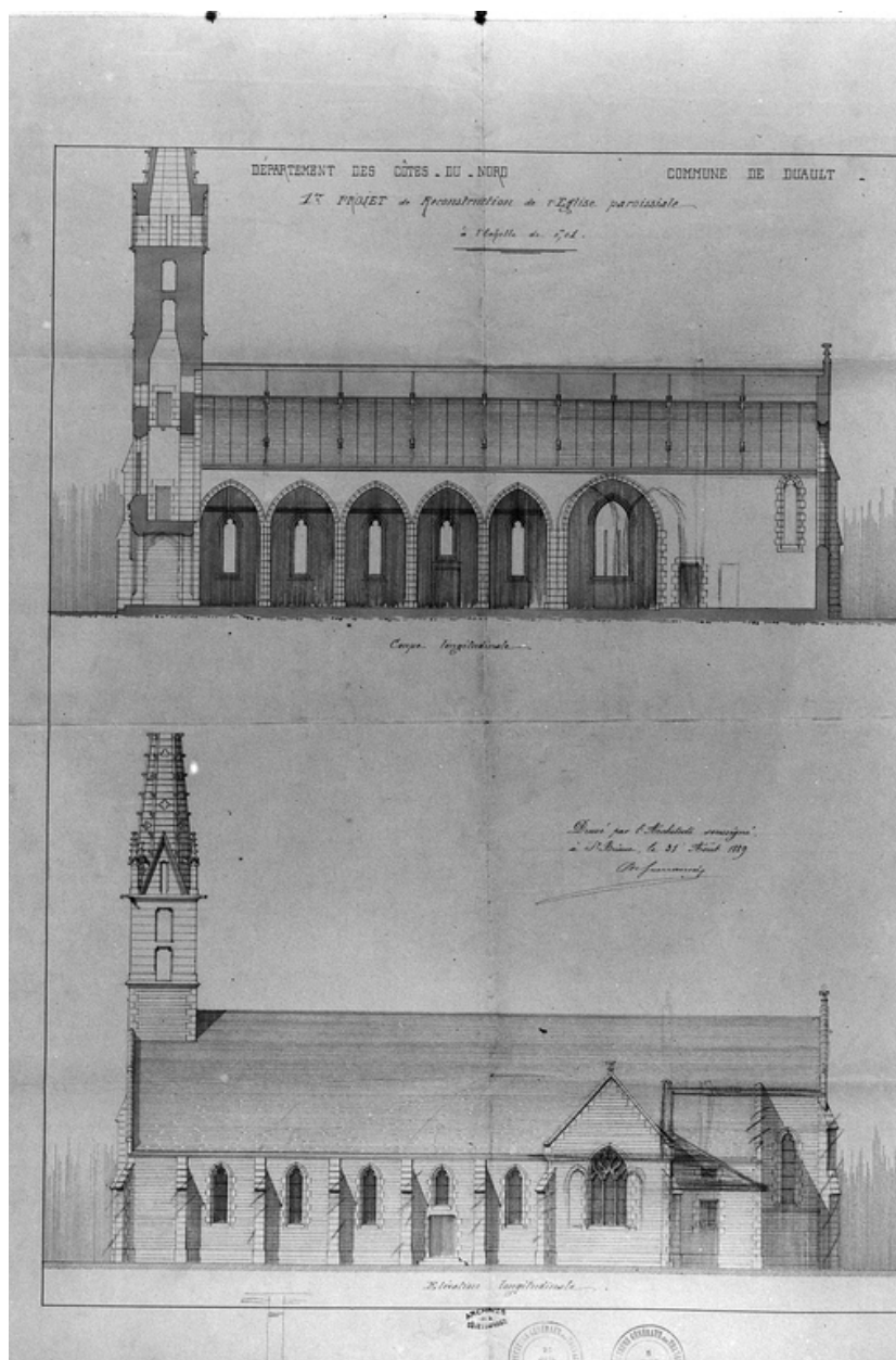
Projets de reconstruction, 1889 (repro. AD Côtes du nord, série V)
