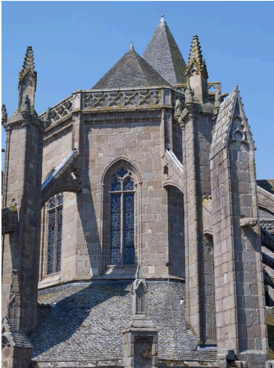
Détail du chevet : pinacles des contreforts
