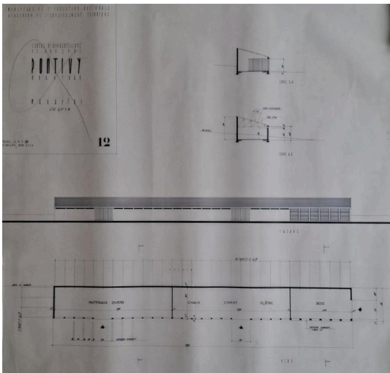
Plan coupes façade des magasins. Yves Guillou, architecte, 1960.
