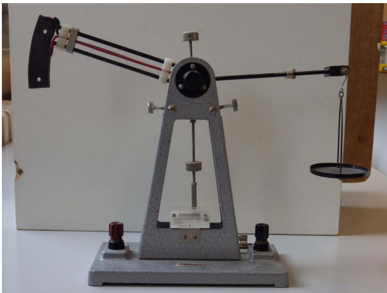
Balance de Cotton - Electricité dynamique (A.O.I.P., deuxième moitié du 20e siècle)
