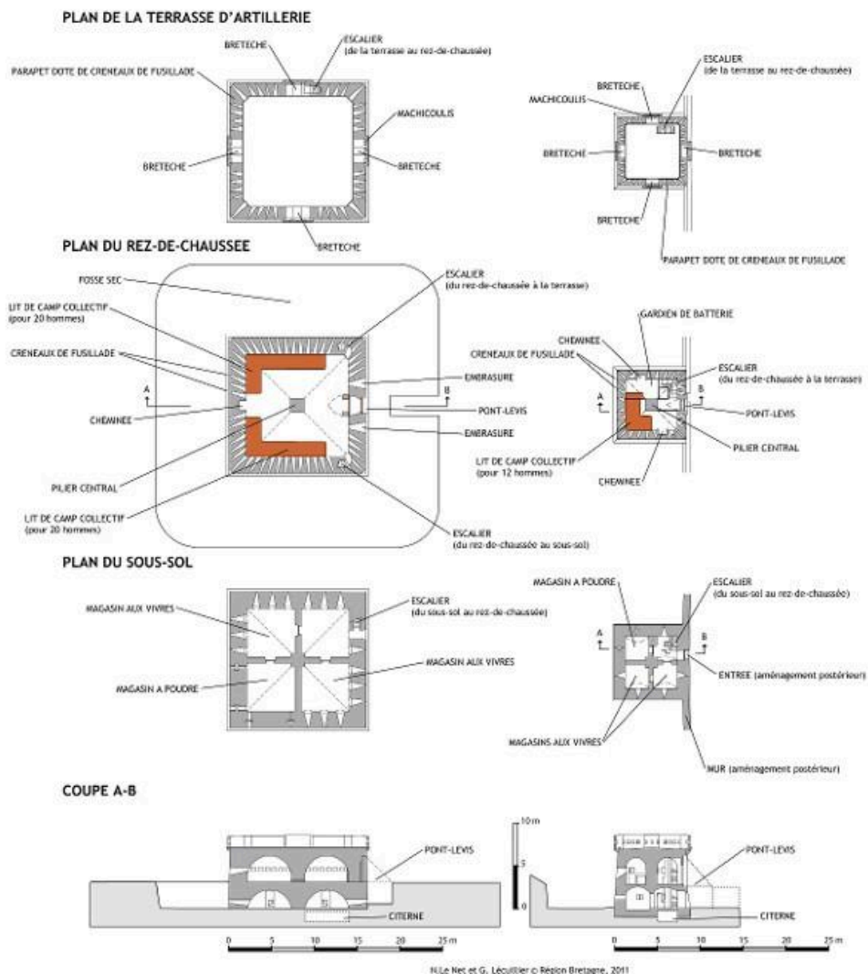
Planche sur les tours-modèles 1811 n° 1 et 3 : plans et coupes
