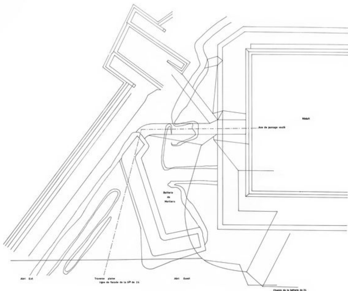
Plan masse entre la batterie de 24 cm et le fort
