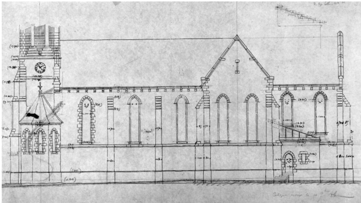
Elévation façade latérale sud. Encre sur calque, 10 sept. 1886, par A. Regnault.
